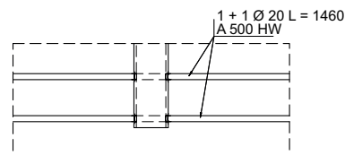
Asennus ontelolaattaan, det 3
